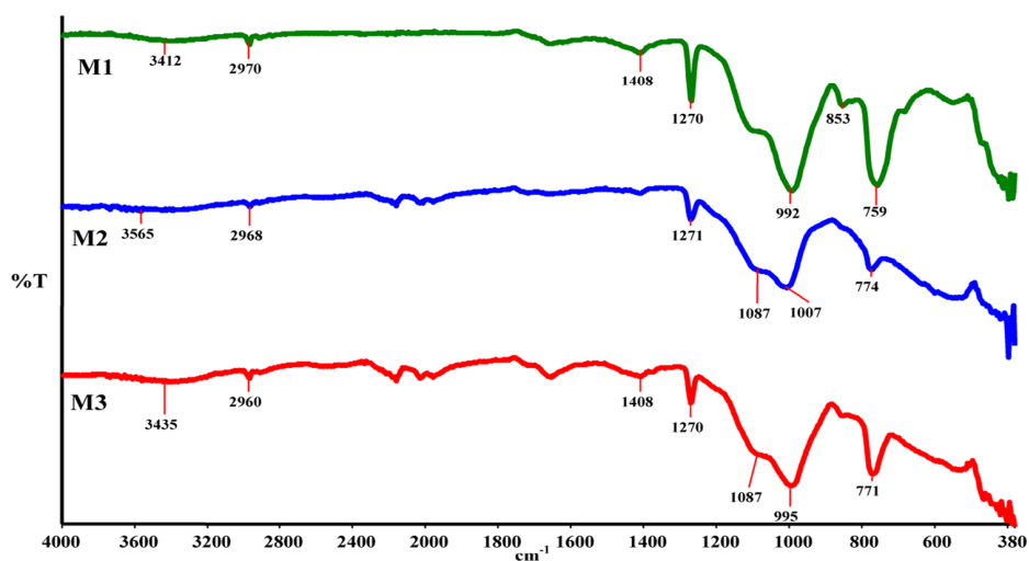
Fig. 5 FTIR spectra of M1, M2 and M3
